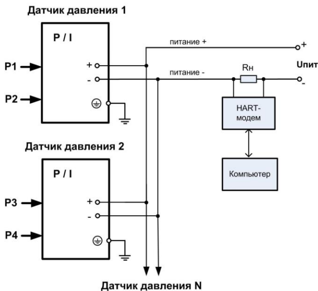
Рисунок В.4 – Подключение нескольких приборов AMZ 5050/AMZ 5450 к одной линии питания (P1–P4 – давление измеряемой среды, R H ≥ 250 Ом)
