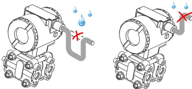
Рисунок 5.4 – Ввод кабеля
