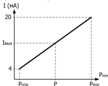
Рисунок В.10 – Характеристики изменения выходного сигнала (тока) от входного давления ( P )
